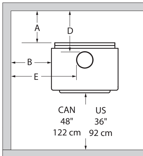
Dégagements - Dessus
