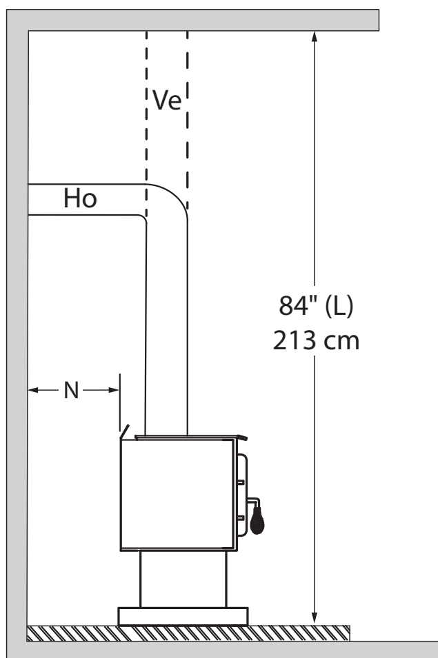
Dégagements - Côté
