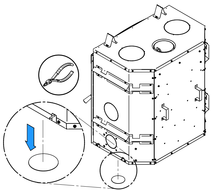
Entrée d'air sous le foyer
